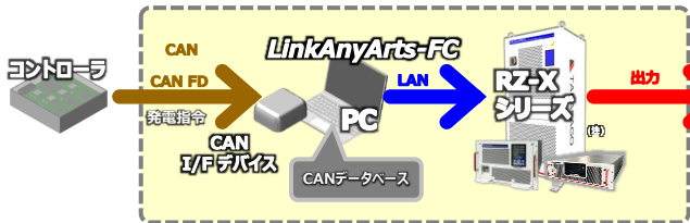
リアルタイムエミュレーションモードの構成
