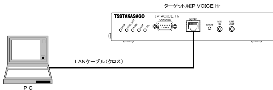
図 9.1
