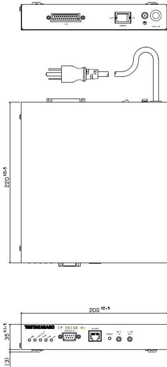
图 10.1 外形寸法图
